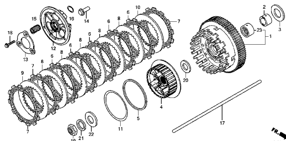
クラッチ (CB1300SADJ, K/SSPK)
